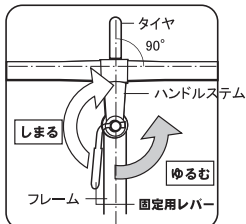
ハンドル部を真上からみた図
